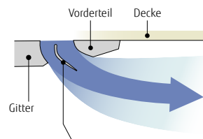
Runde Lamelle
