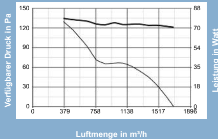
A-E 304T - 42227
