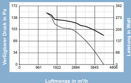
A-E 404M - 42260
