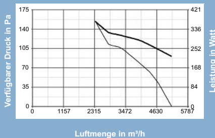
A-E 454T - 42308
