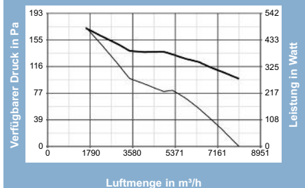
A-E 566T - 42366
