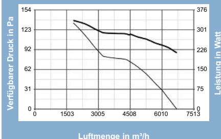
A-E 566M - 42356
