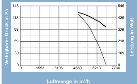
A-E 504T - 42327
