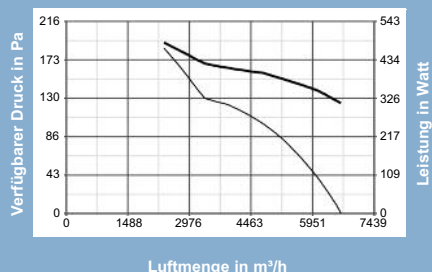
A-E 504M - 42316
