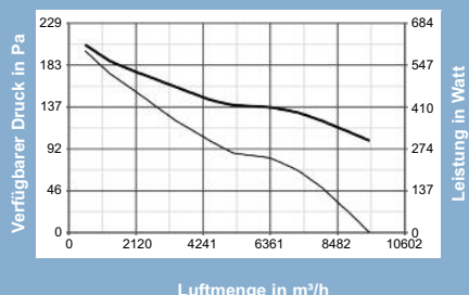
A-E 636T - 42347
