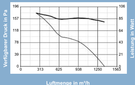
A-E 252M - 42207
