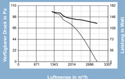
A-E 354M - 42258
