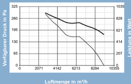
A-E 564T - 42336
