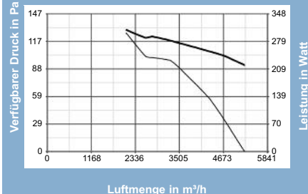
A-E 454M - 42307
