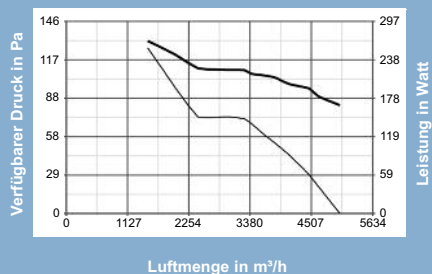
A-E 506T - 42346
