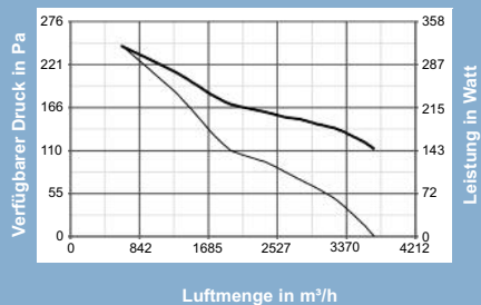
A-E 404T - 42261
