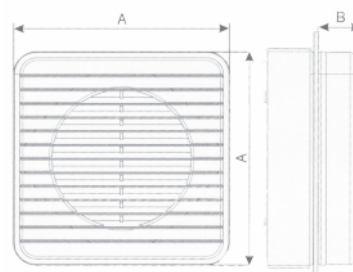
Abmessungen FK ín
