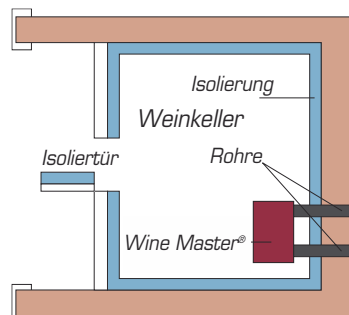
Installationsschema für C50INX
