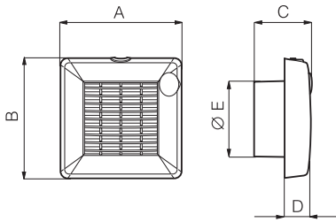
Abmessungen Serie Punto
